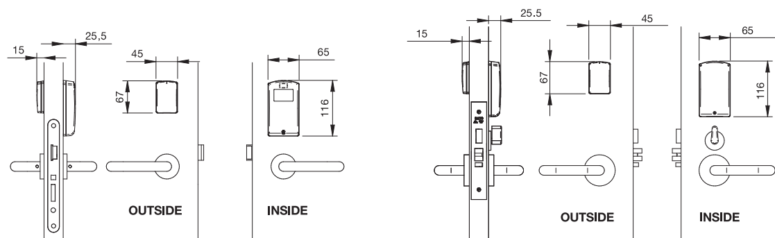
Modelo LE7E37 estándar DIN
