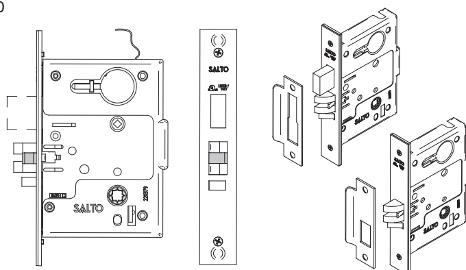
Modelo LA1M1770 estándar ANSI
